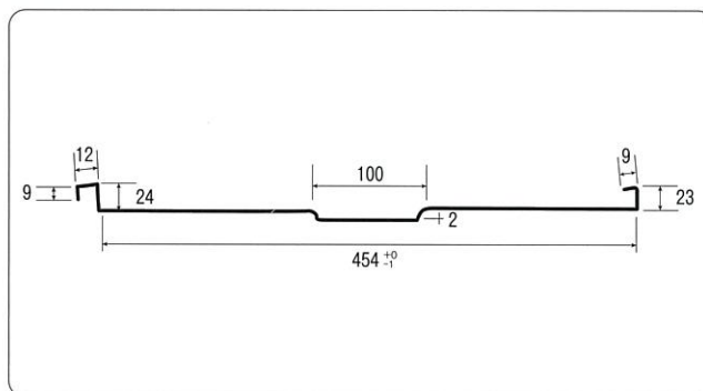
断面形状図
