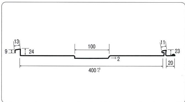
断面形状図
