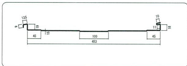
断面形状図
