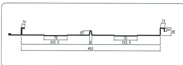
断面形状図
